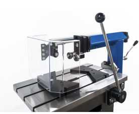
Kryt drážkovačky DR 050
